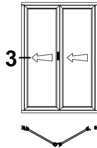
Section 3: Jamb
